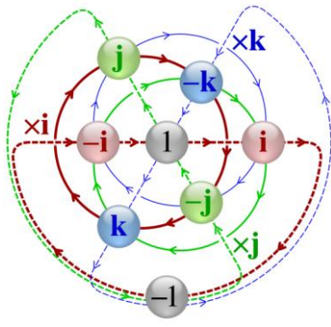
Рисунок 1 – Кватернион
